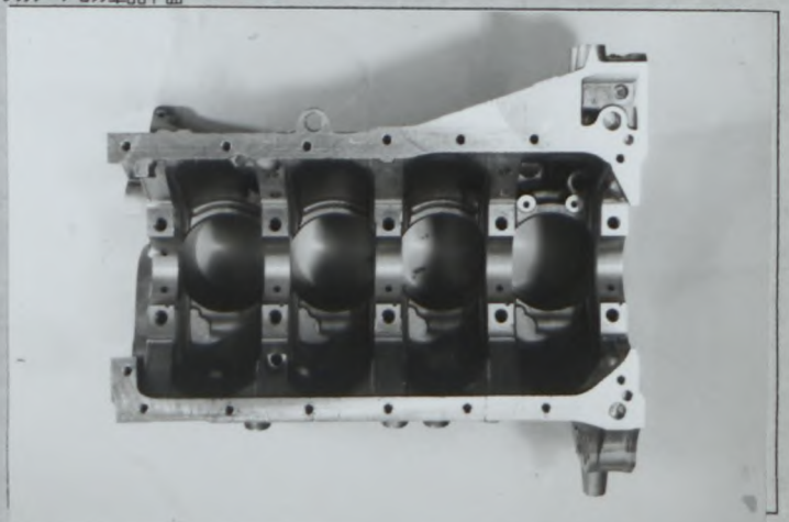
Profil gauche du bloc nu Left hand view of bare block シリンダブロック単品左側面
