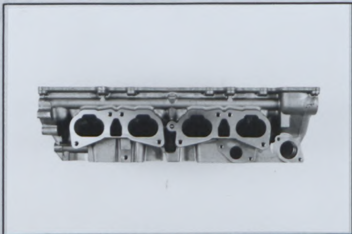
Profil droit de culasse nue Right hand view of bare cylinderhead シリンダ-ヘッド単体の右側面
