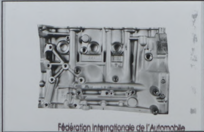
Profil gauche du bloc nu Left hand view of bare block ブロック単体の左側面
