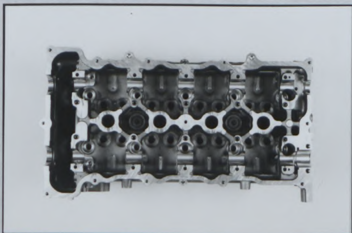
Culasse nue vue de dessus Bare cylinderhead seen from above シリンダ-ヘッド 単体の上面視
