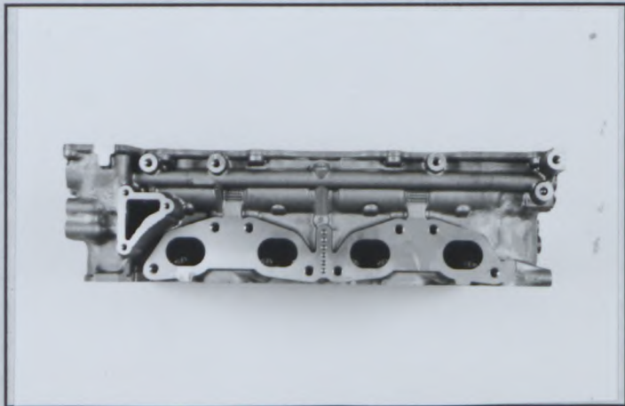
Profil gauche de culasse nue Left hand view of bare cylinderhead シリンダ-ヘッド単体の左側面
