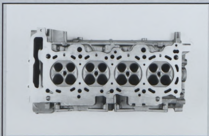
Culasse nue vue de dessous Bare cylinderhead seen from below シリンダ-ヘッド 単体の下面視
